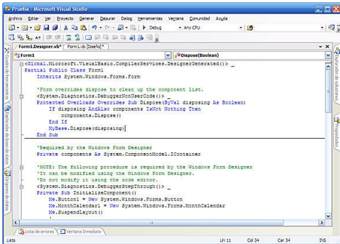
Figura 1.5.- Código autogenerado por Visual Studio para crear la interfaz de la figura anterior.
