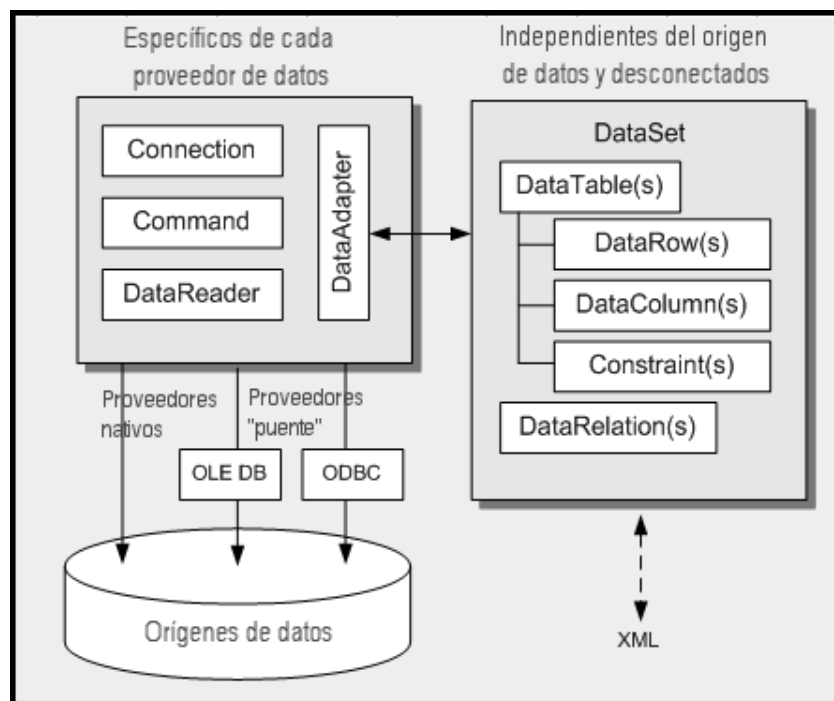
Figura 1.3.- Arquitectura de ADO.NET
